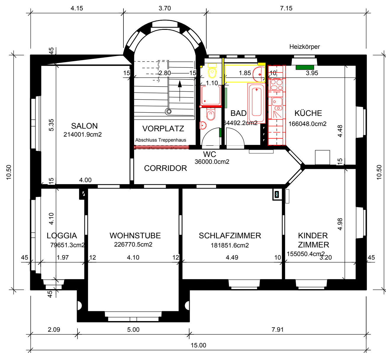
HOCHPARTERRE 1: 100
