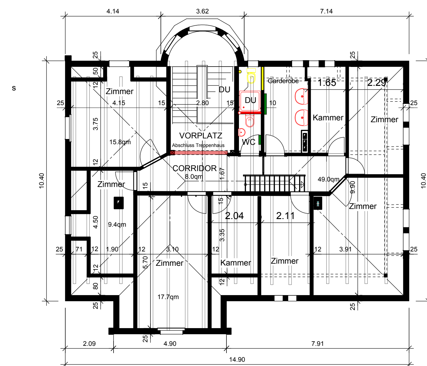
DACHGESCHOSS 1: 100
