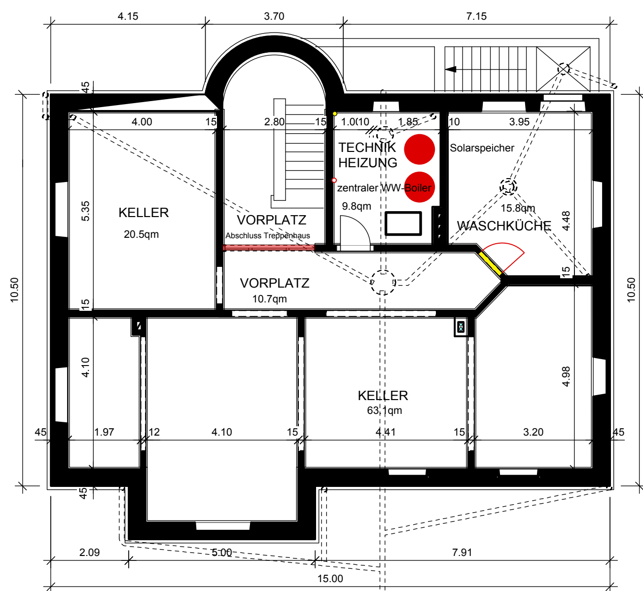
KELLER 1: 100
