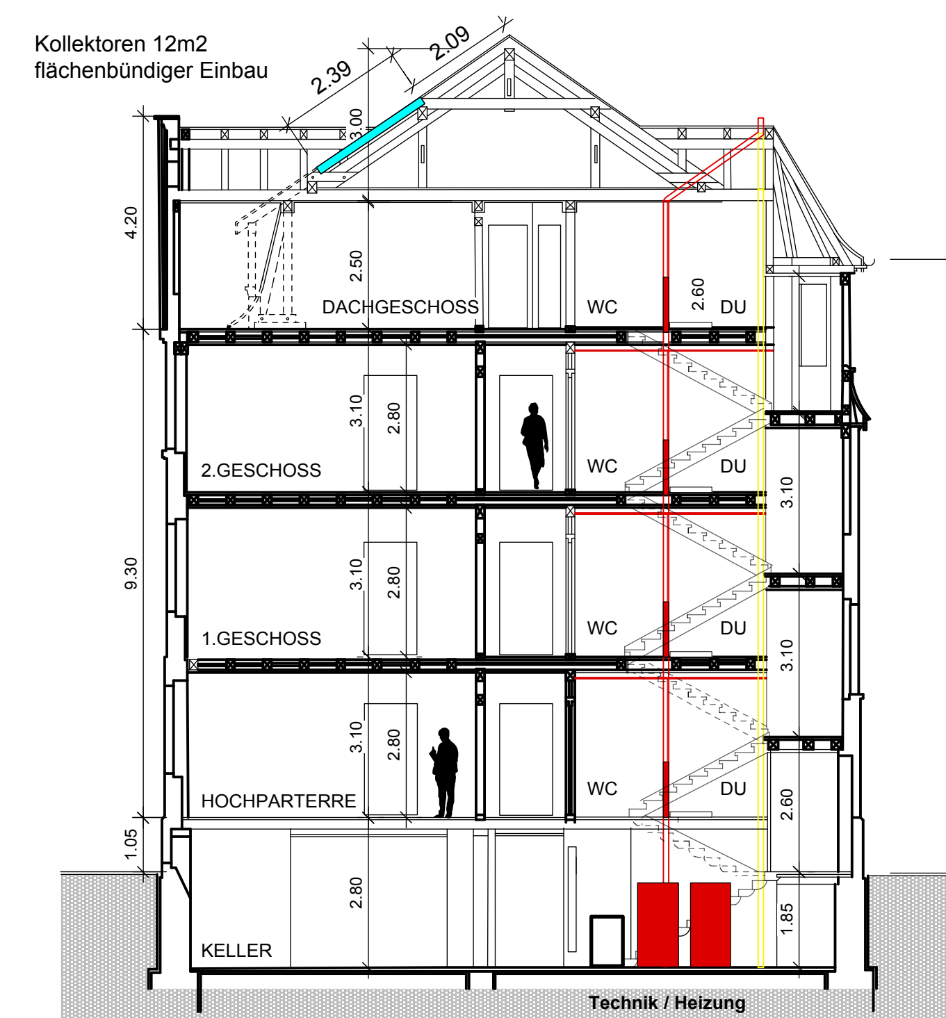
QUERSCHNITT 1: 100
