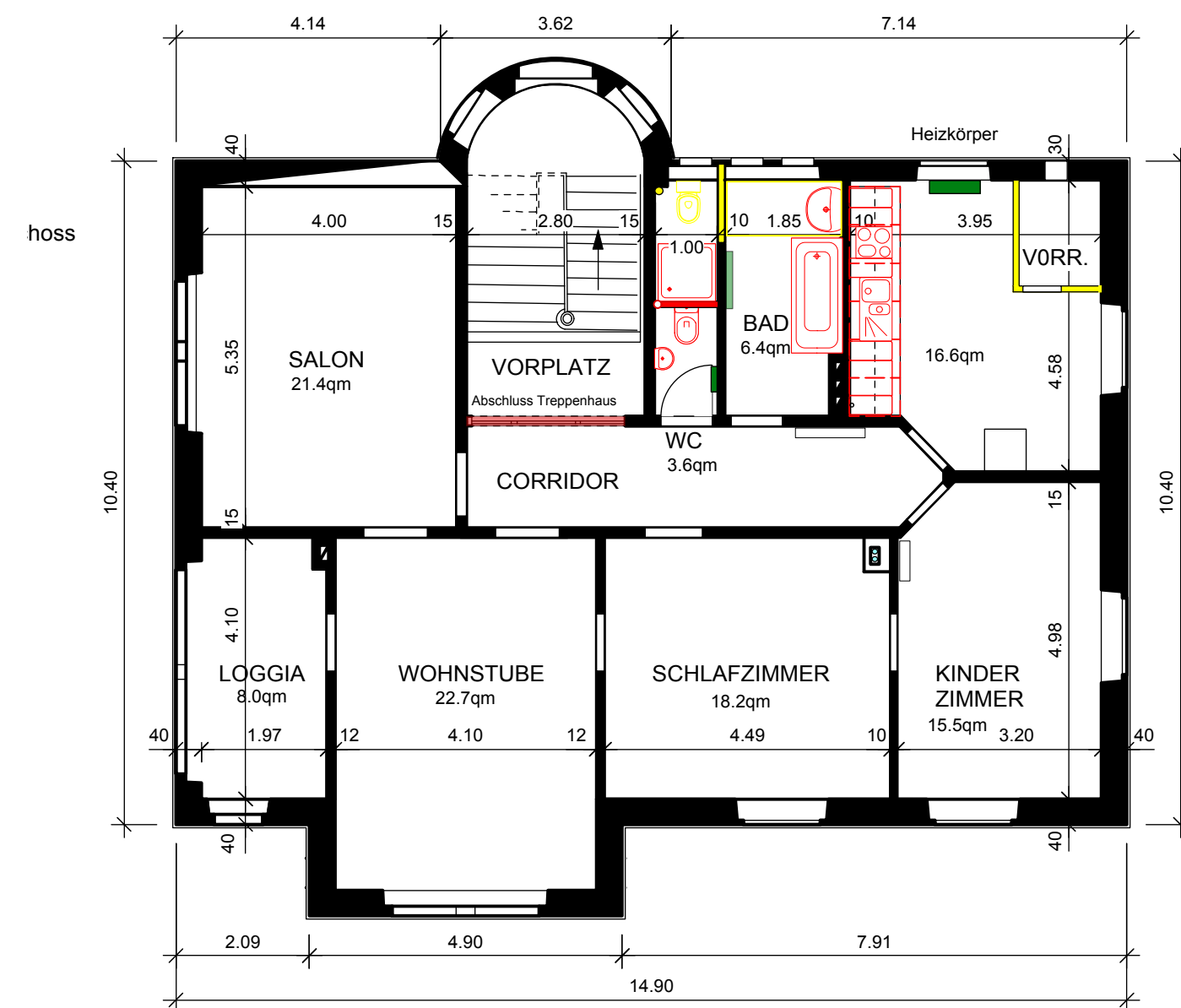
1.- UND 2. GESCHOSS 1: 100
